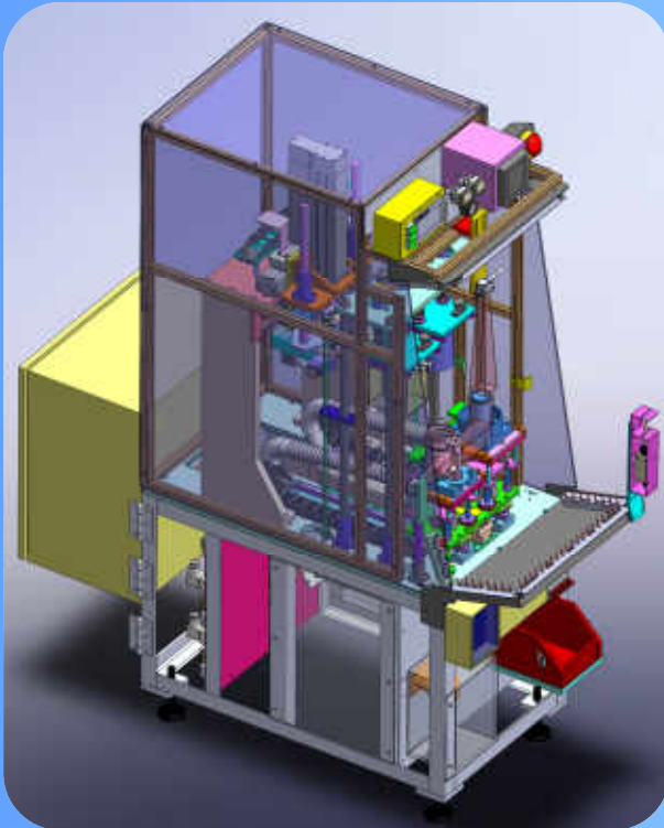
Servo Press
