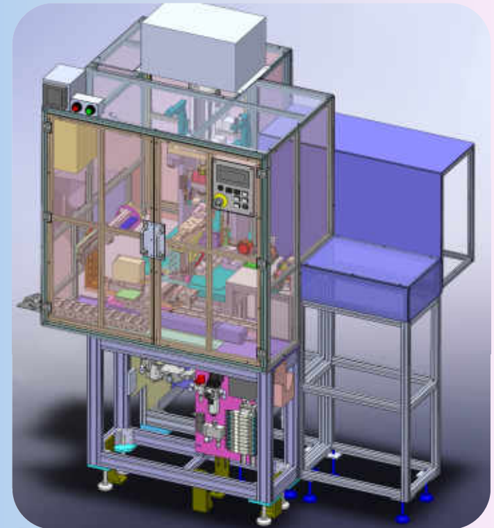
Air Hydro Press +Loader Auto
