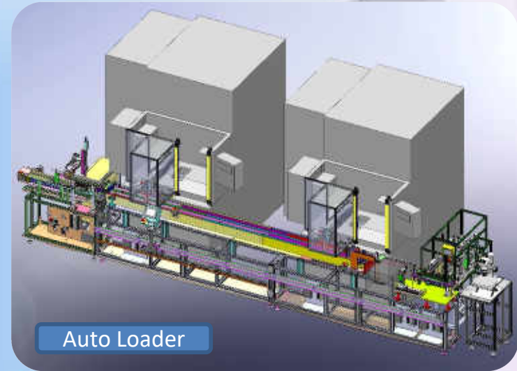
Auto Loader
