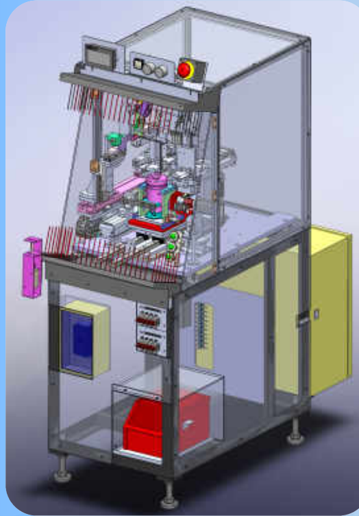
Tube Press
