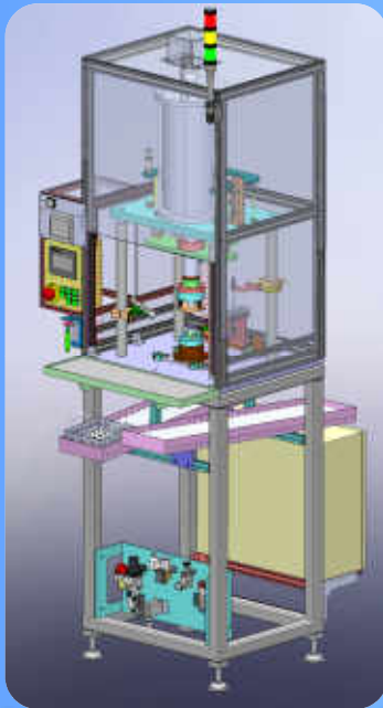
Air Hydro Press
