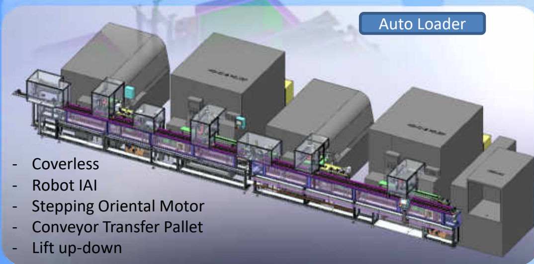
Auto Loader
